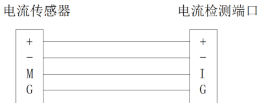
图六 电流传感器接线示意图
