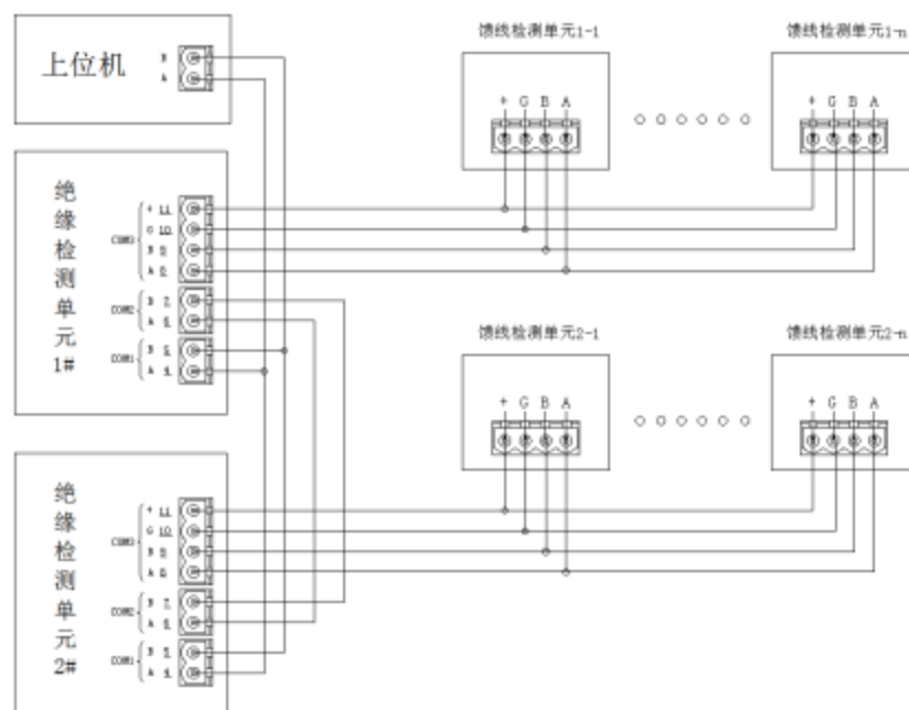
接线示意图
