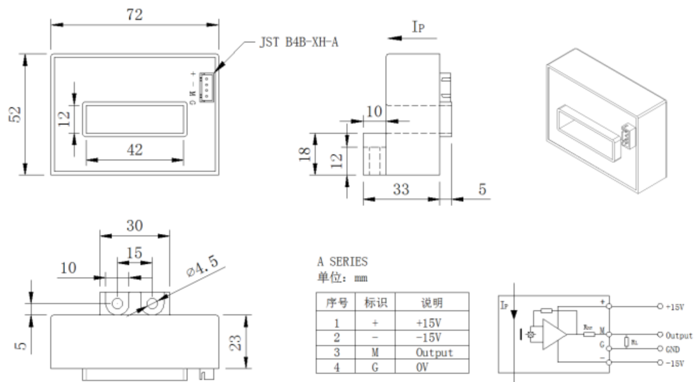
SCK4A 外形尺寸
